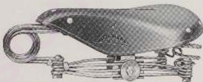
214 la starker Hammocksattel mit dreifacher Brücke, gedrillten hinteren Spiralen und doppelt gewundener Vorderfeder. Ledergröße 30 \times 26 cm. la Kernleder
