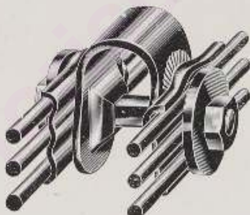
Kloben für 3-Feder-Sattel
