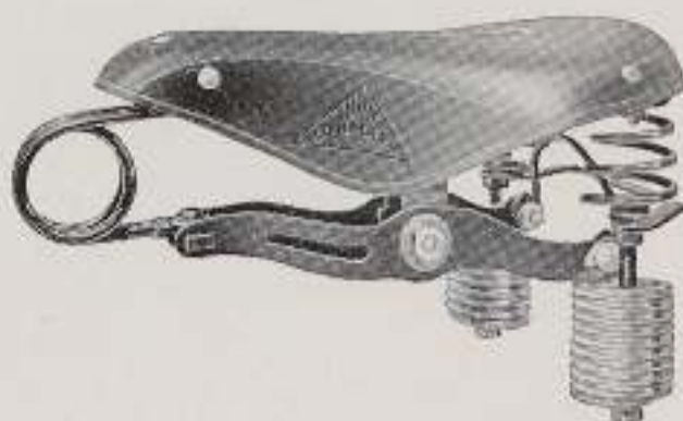
215 Extra starker großer Sattel mit Schiene, Zug- und Druckfedern und Vorderfeder. Außerordentlich beliebtes Modell! Ledergröße 30 \times 26 cm
