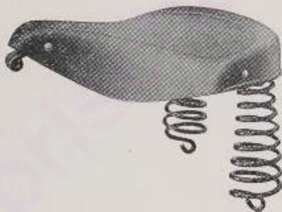
275 y Motorradsattel für Dreipunktaufhängung mit bester Spezial-LOHMANN-Gummidecke mit Sportkante
